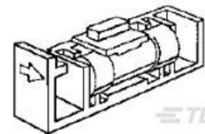
TE 系列/零件编号1609144-1 LA200 DL US FUSEHOL=F6927
