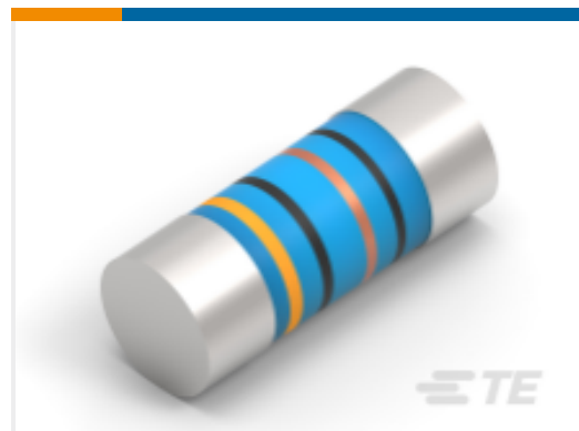
TE 系列/零件编号8-2176315-2 MELF SMA-A 39R 1% 50PPM 0204 0.4W
