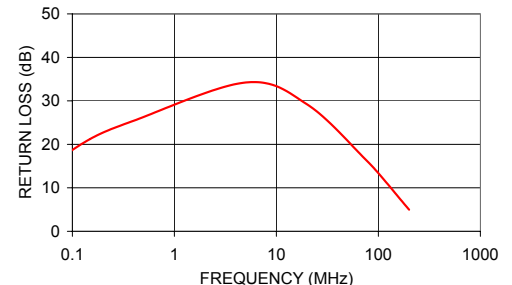
TMO-4-6+ INPUT RETURN LOSS
