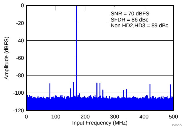
170MHz 输入信号的 FFT
