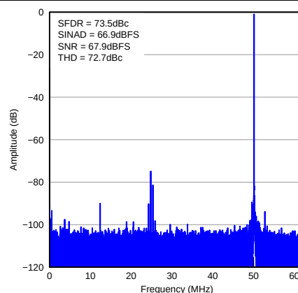
图 89. FFT for 300-MHz Input Signal
