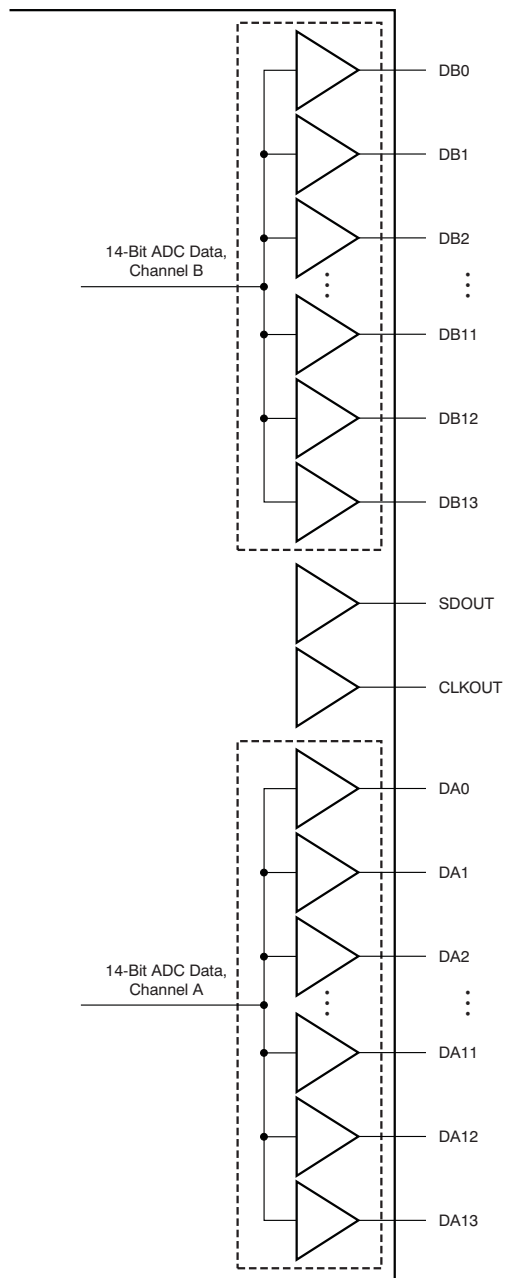
图 158. CMOS Outputs
