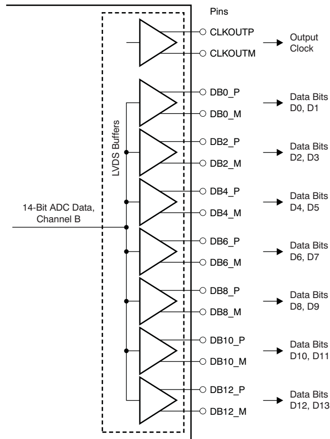
图 154. LVDS Interface
