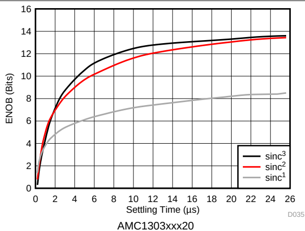
图 53. 测得的有效位数与建立时间间的关系
