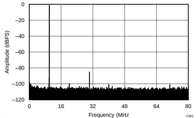
启用抖动功能时的快速傅立叶变换 (FFT) ( f_s = 160\text{MSPS} , f_{IN} = 10\text{MHz} , SNR = 70.3dBFS, SFDR = 84dBc)
