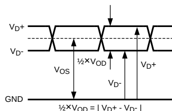
图 59. LVDS 输出信号电平
