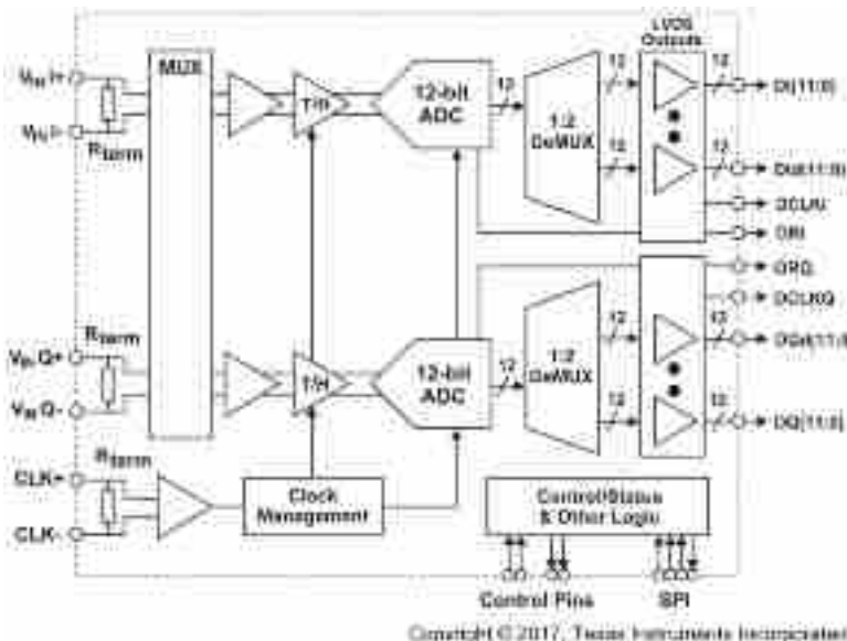
功能框图
